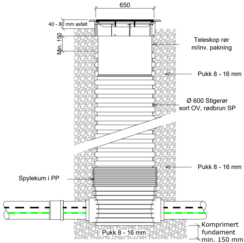
SNITT A - A
