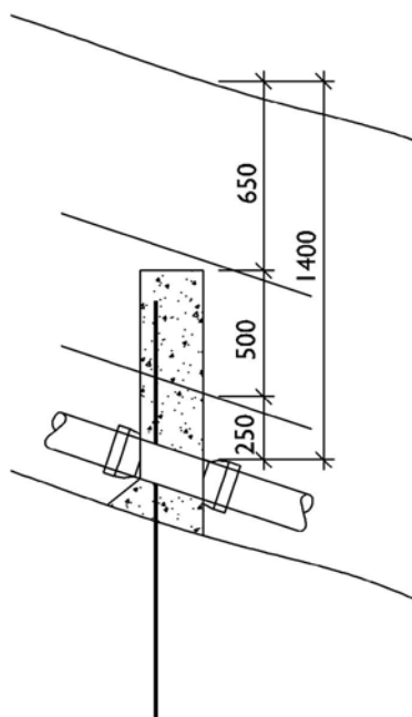
Lengdesnitt
