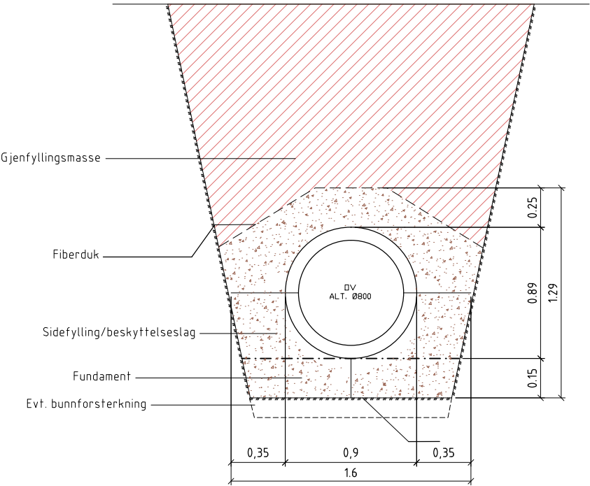
Grøftesnitt ikke i målestokk
