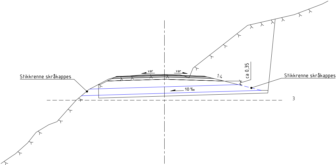
Normalprofil Skjæring - detaljer stikkrenne
