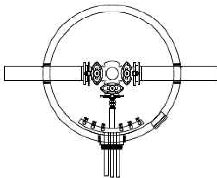
Løsning med manifold
