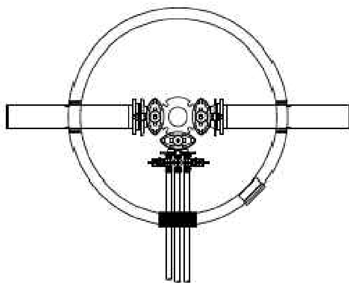
Løsning med koblingsflens tilpasset inntil 6 stikkledninger
