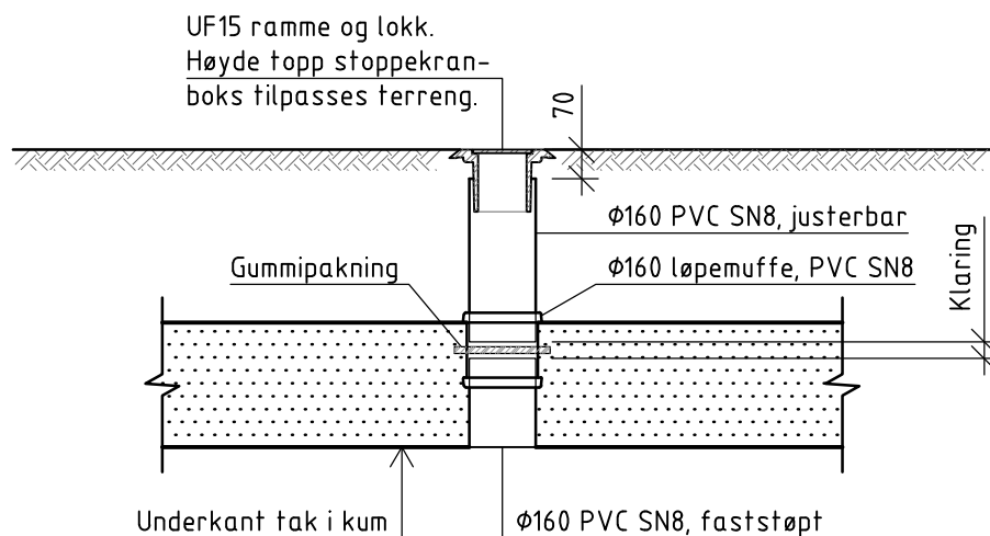
Detalj av gategutt/stoppekranboks med innstøpt løpemuffe
