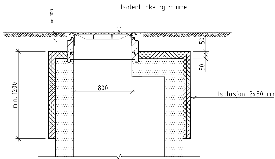
SNITT A-A
