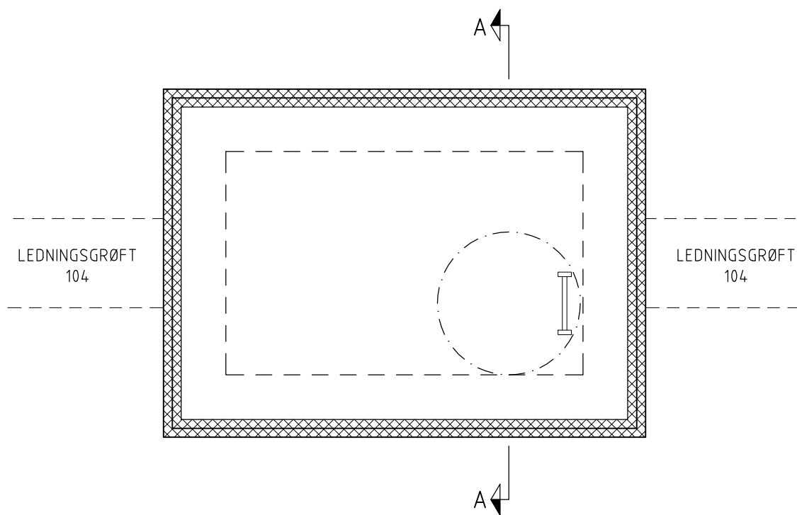
PLAN PLASSTØPT FIRKANTKUM MED ISOLASJON
