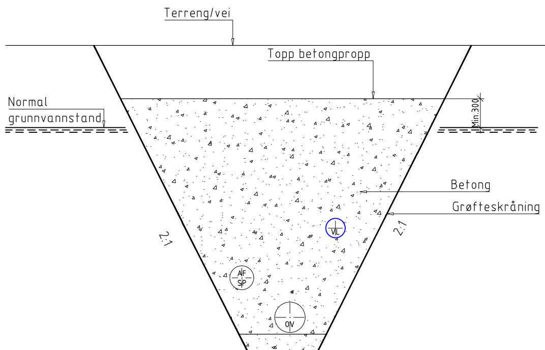
SNITT A-A - BETONGVEGG
