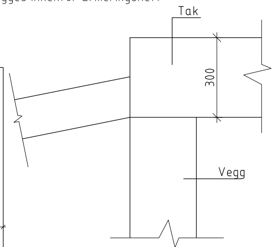
DETALJ 2 VED KUMVEGG
