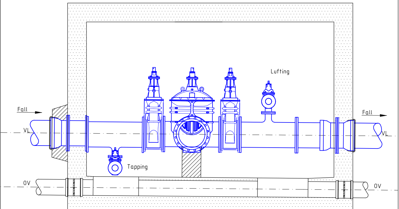
SNITT A - A
