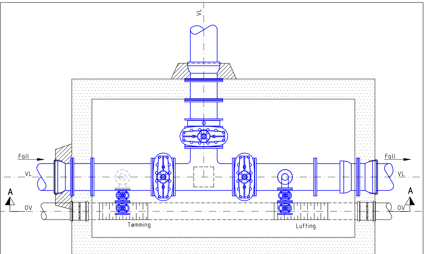
PLAN ENSIDIG FALL PÅ OVERFØRSELSESLIEDNING
