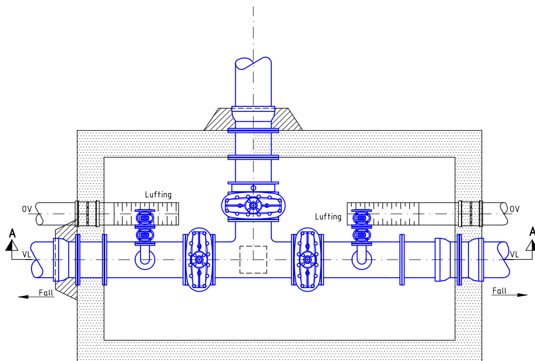
PLAN HØYDEBEPUNKT PÅ OVERFØRSELSESLIEDNING
