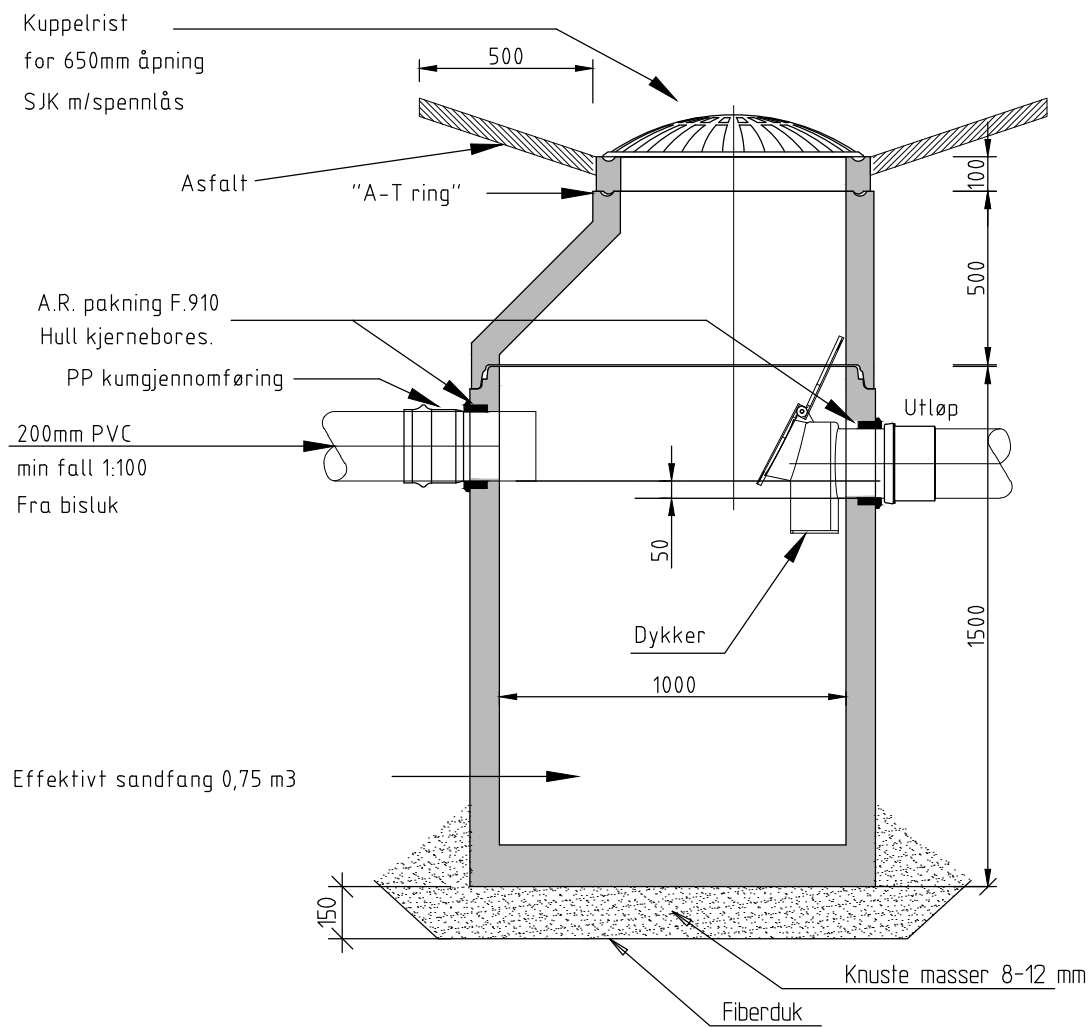
SNITT A-A
