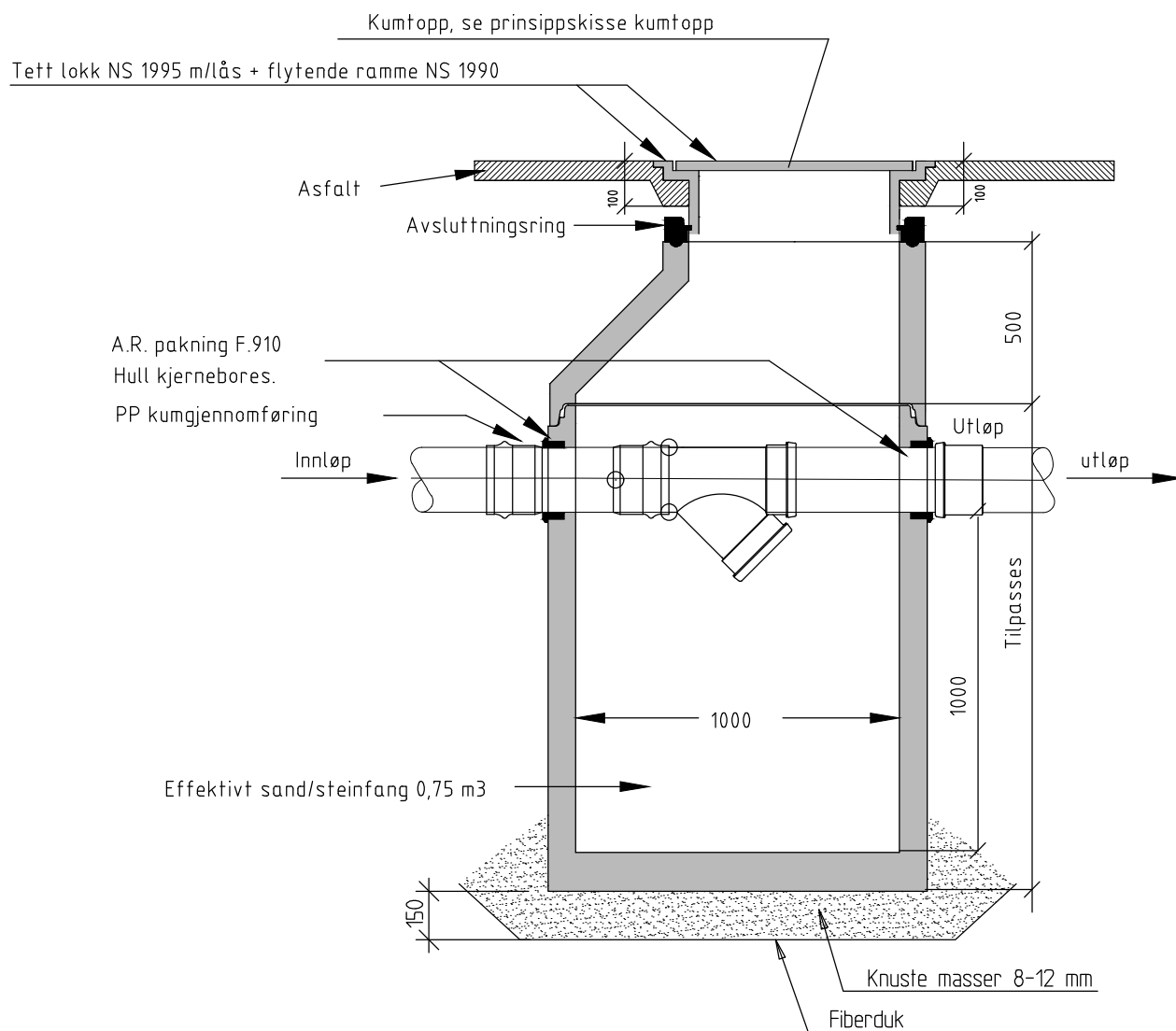
SNITT A-A
