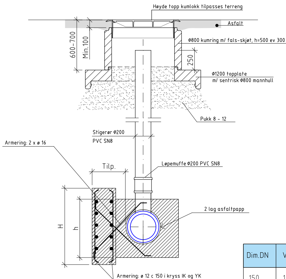
Snitt A-A, forankring bend og markeringskum
