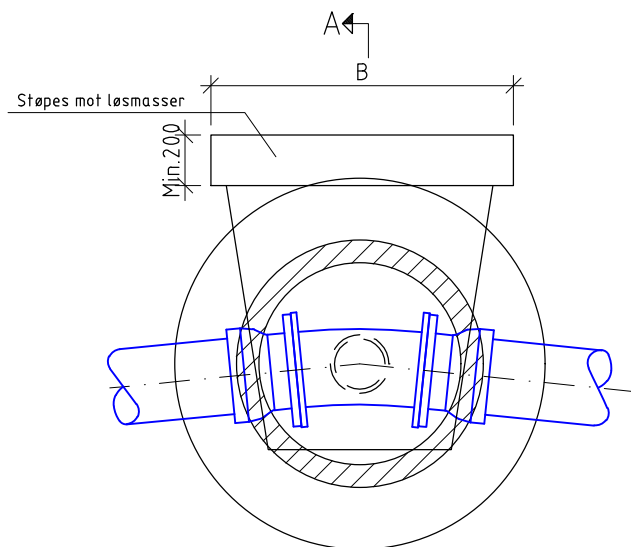
Forankring av bend på vannledning i jord-grøft
