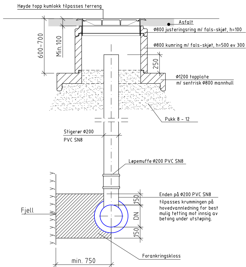
Snitt B - B
