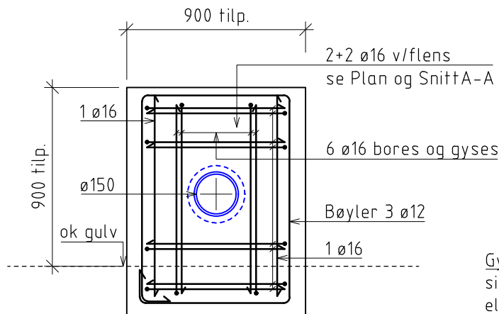
SNITT B-B
