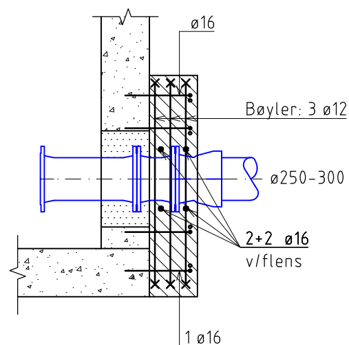
SNITT A-A
