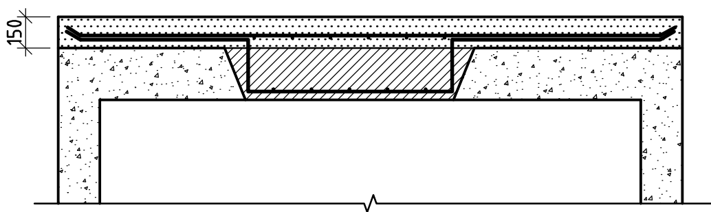
SNITT A-A
