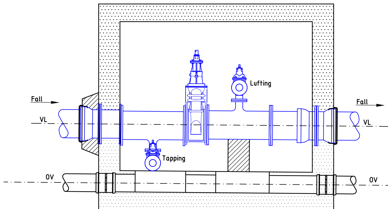
SNITT A - A
