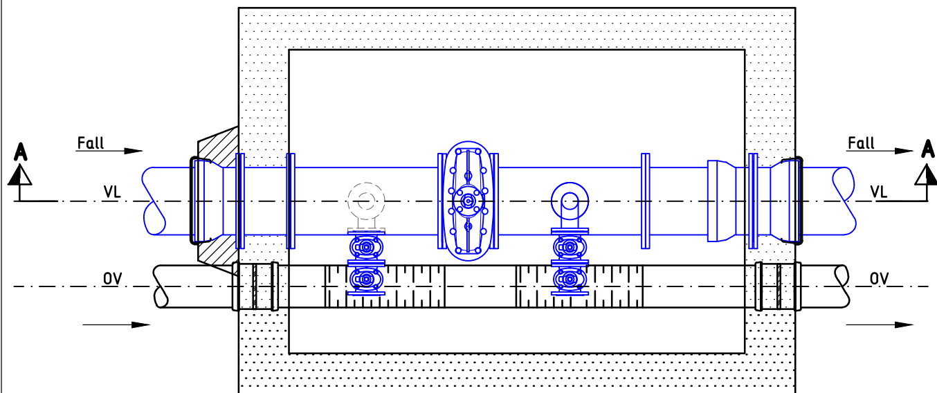
PLAN ENSIDIG FALL PÅ OVERFØRSELSESLEDNING
