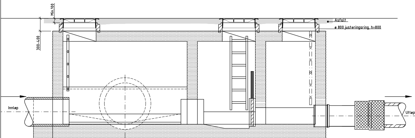
OVERLØPSKUM SNITT
