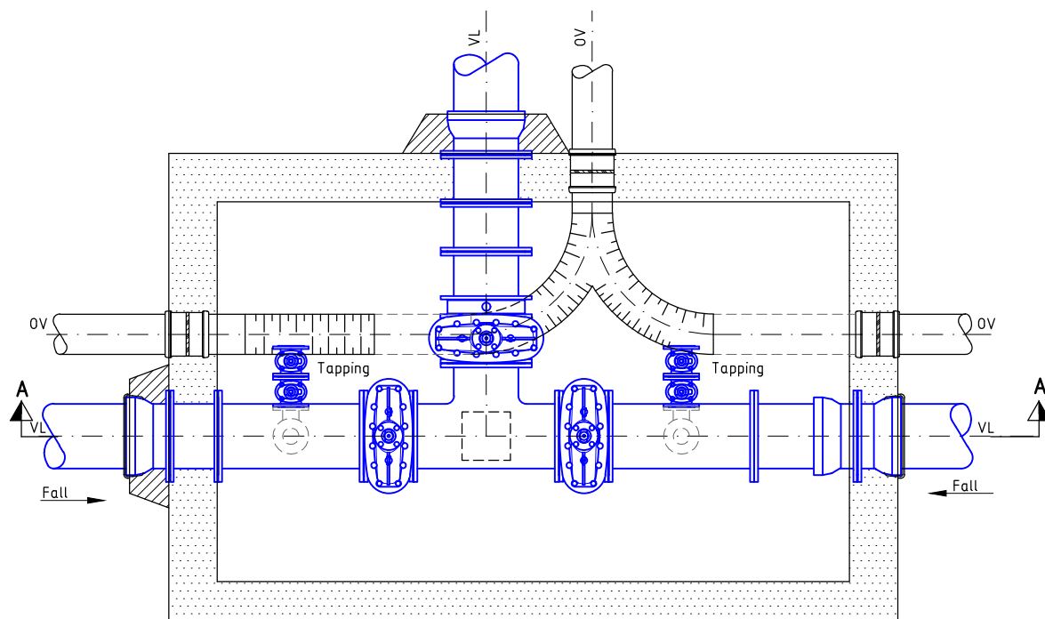
PLAN LAVPUNKT PÅ OVERFØRSELSESLIEDNING
