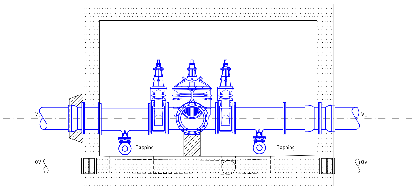
SNITT A - A
