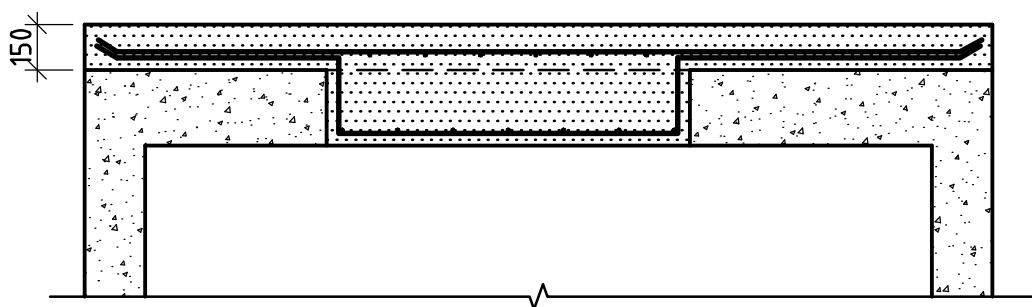
SNITT A-A
