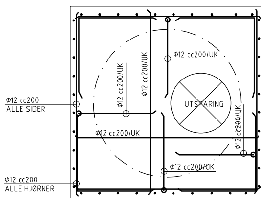
PLANSNITT A-A
