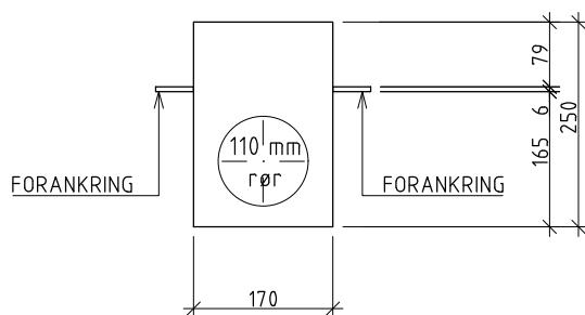
SNITT B-B
