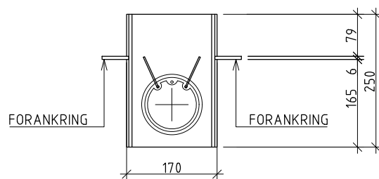
SNITT C-C
