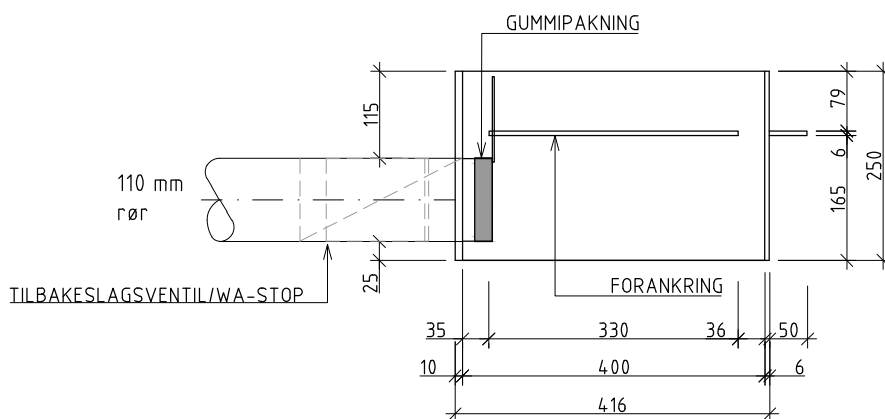
SNITT/OPPRISS A-A
