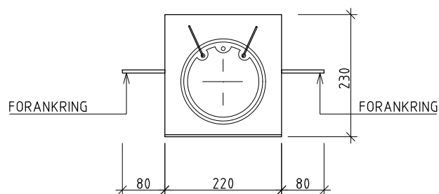
SNITT C-C
