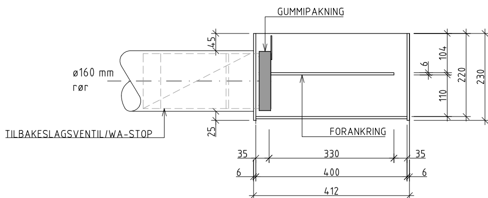
SNITT/OPPRISS A-A
