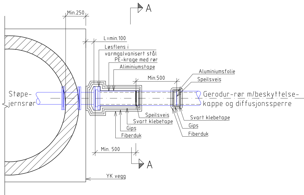
Gerodur-skjøt utvendig kum m/speilsveis
