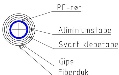
Snitt A-A PE-krage med Gerodur rør
