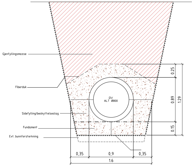
Grøftesnitt ikke i målestokk
