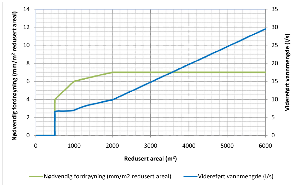
Figur2: Separatsystem. Minimumskrav til fordrøyning og maks videreført vannmengde.
