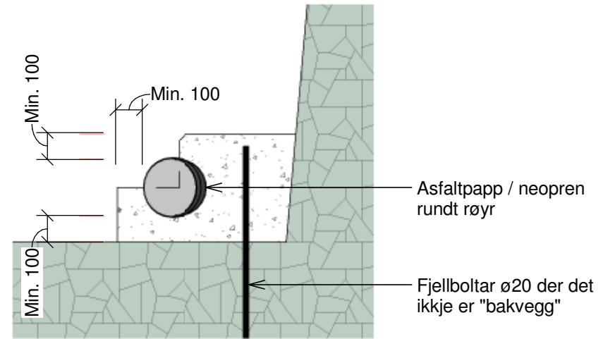
SNITT
