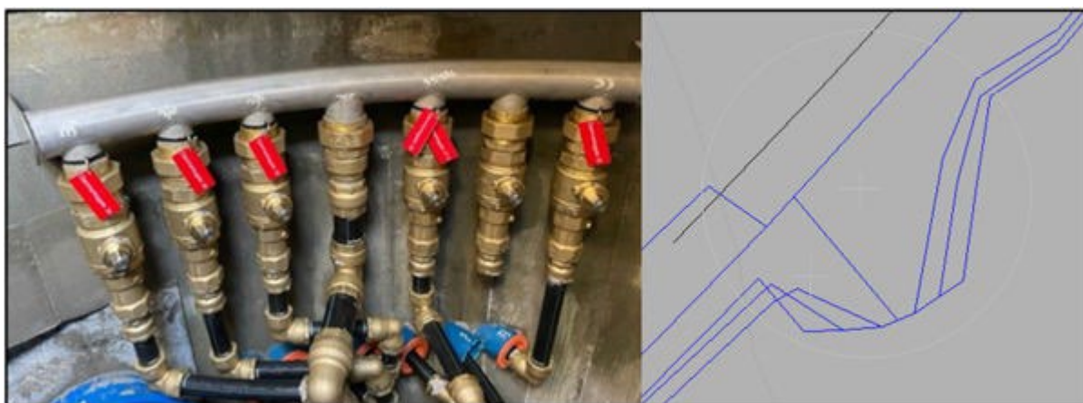
Figur 8. Innmåling av stikkledninger gjennom manifold.
