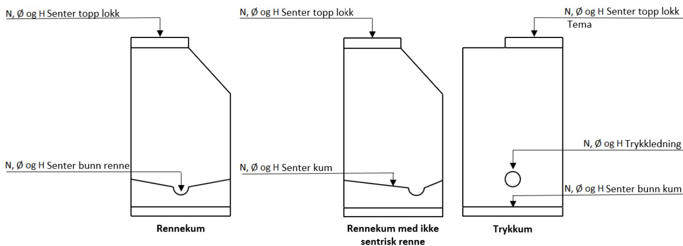
Figur 10. Hvordan måle inn konstruksjon med lokk.
