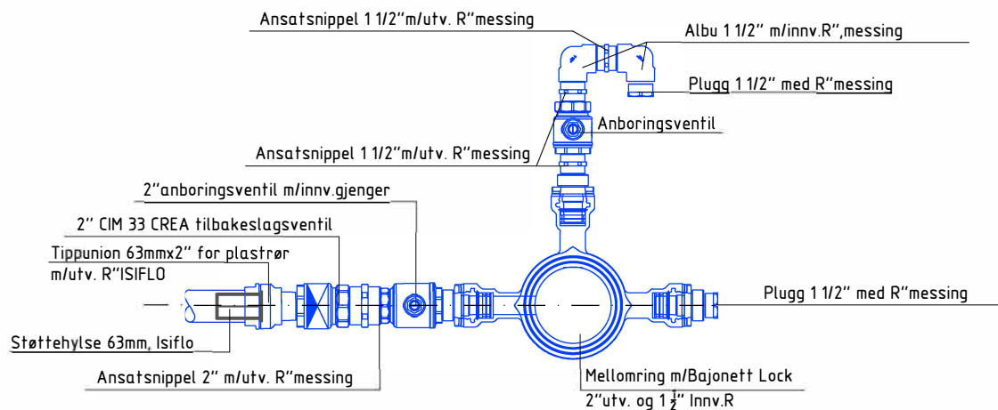
Stikkledning 63 mm på mellomring (med mulighet for trykkprøving, kloring, lufting)
