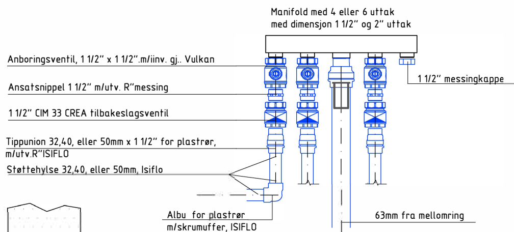
Fra samlestock til stikkledninger
