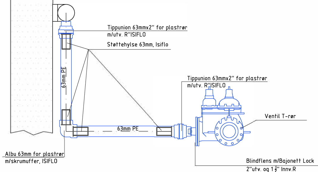
Fra mellomring til standard manifold
