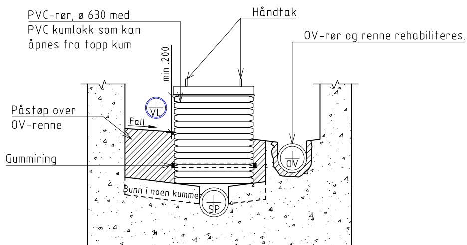
SNITT A-A
