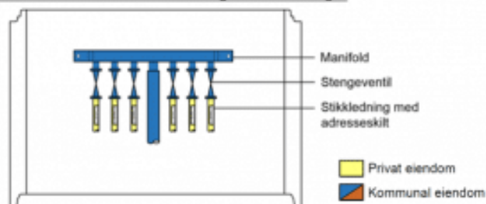
Grensesnitt i vannkum for fordeling av stikkledninger
