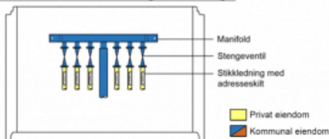
Grensesnitt i vannkum for fordeling av stikkledninger
