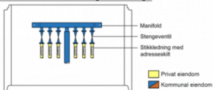
Grensesnitt i vannkum for fordeling av stikkledninger
