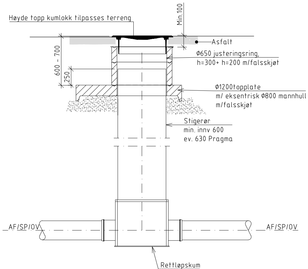
Snitt
